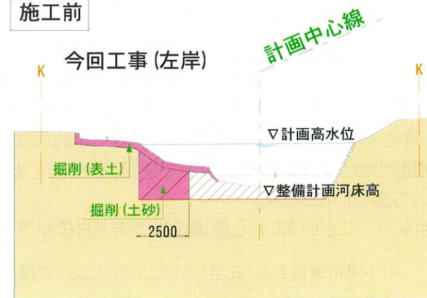
標準断面図
